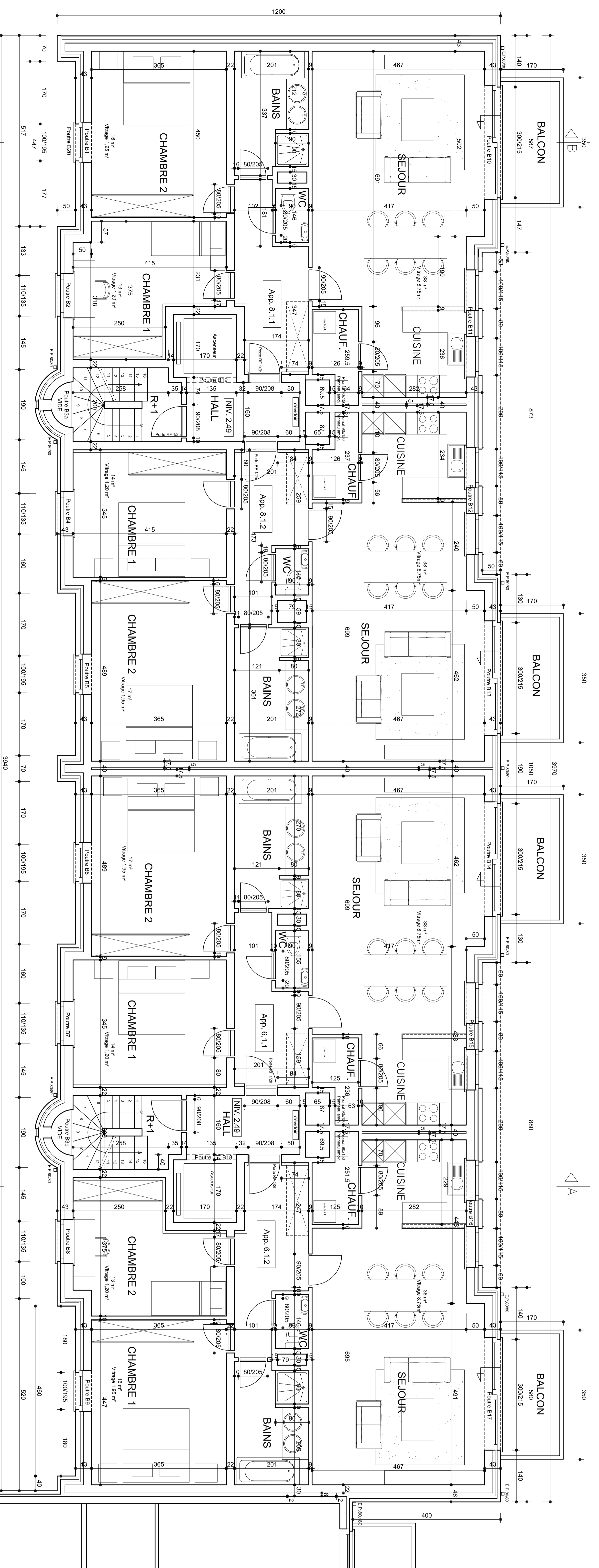
PLAN ETAGE 1
